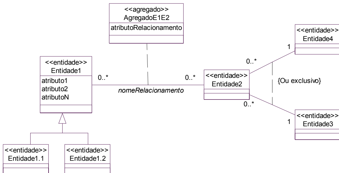
Figura 5.49 – Diagrama ER usando a notação da UML.
