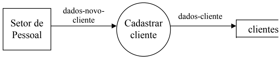
Figura 5.32 – Mesmo conteúdo de dados em fluxos diferentes.
