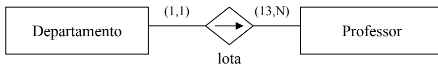
Figura 5.6 – Representação de cardinalidades em relacionamentos.
