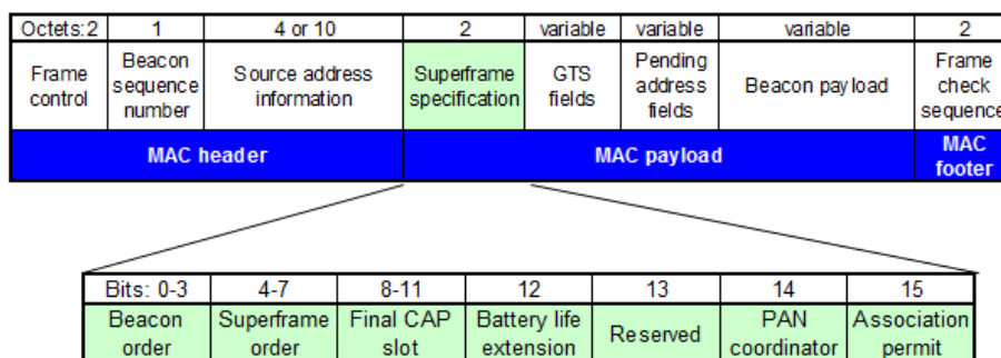
Figura 16 – Formato do Quadro Beacon
