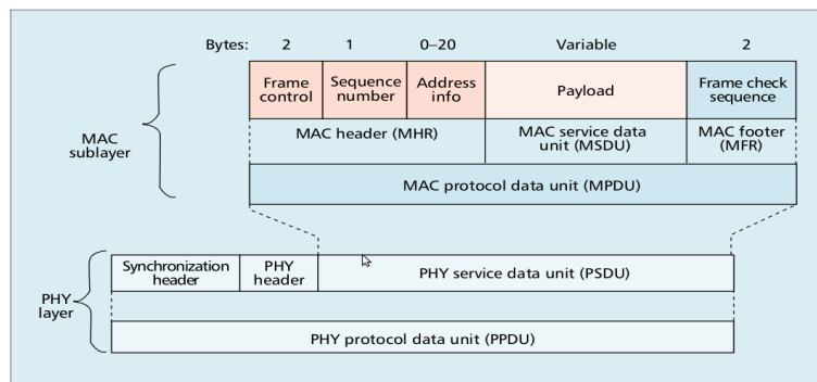
Figura 13 – Encapsulamento de uma MAC PDU na Camada Física
